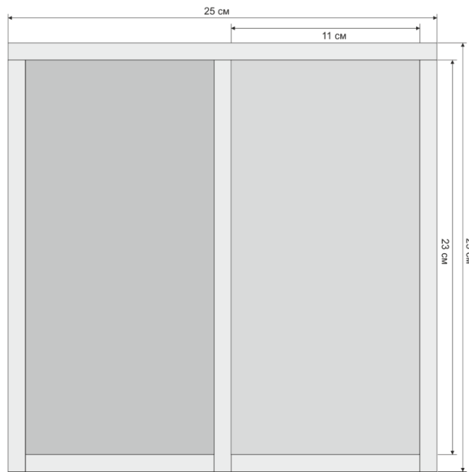
Приложение 3. Элемент двускатный
